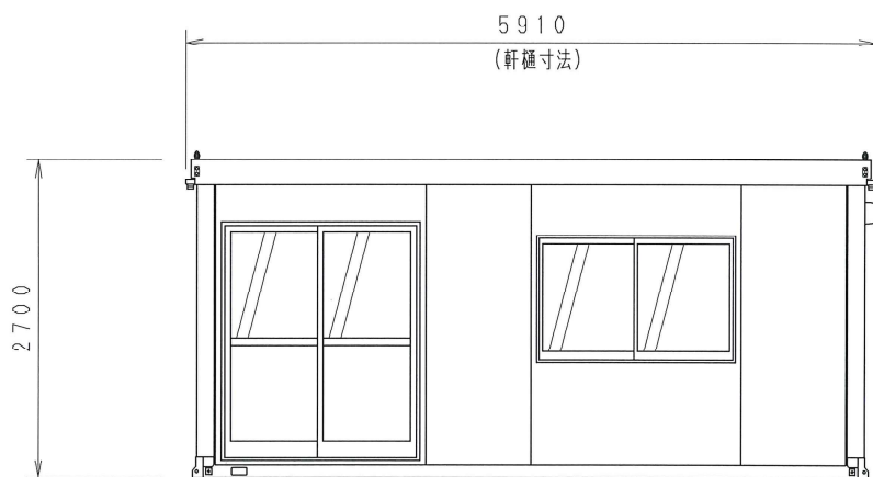
A 立面図
