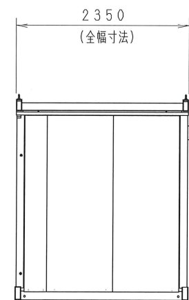
D 立面図
