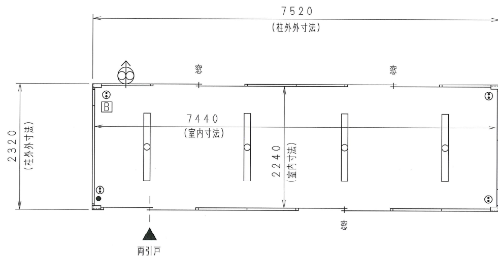
平面図
