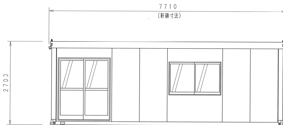
A 立面図
