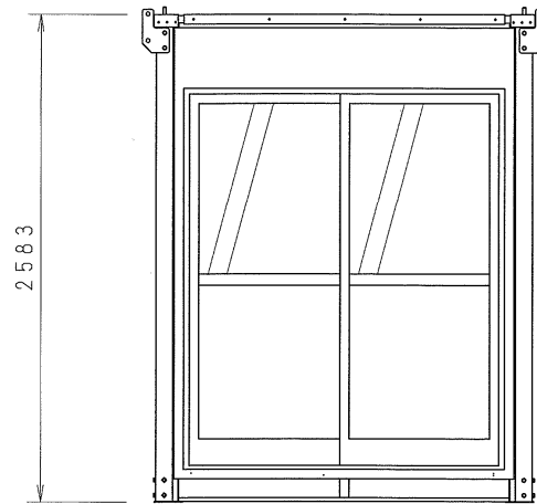
A 立面図
